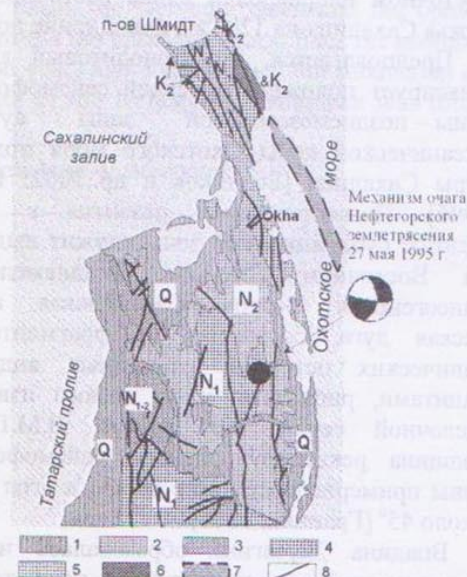
Рис. 1. Геологическая карта Северного Сахалина. Механизм очага Нефтегорского землетрясения дан по [2].
