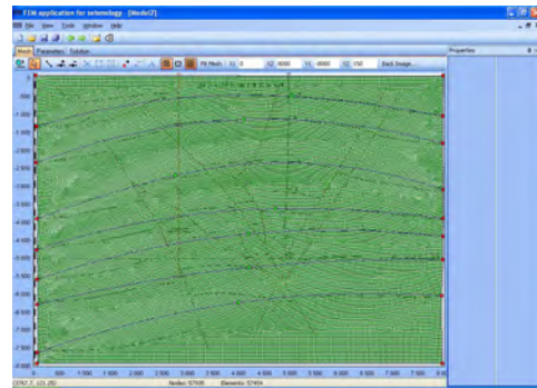
Рис.2 Модель шаруватого середовища побудована за геофізичними та сейсмічними даними
