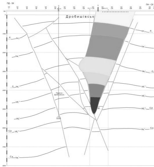
Рис.7 Виділена ділянка перетину Дробишівської площі моделювання МСЕ.
