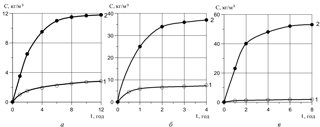
Рис. 1. Кінетичні залежності процесу екстрагування олії хлористим метиленом з насіння амаранту гібриду (а); ріпаку (б); рижію (в) за температури 30 °С: 1 – із неподрібненого насіння; 2 – із подрібненого насіння з фракцією d_{сер} = 0,25 \cdot 10^{-3} \text{ м}
