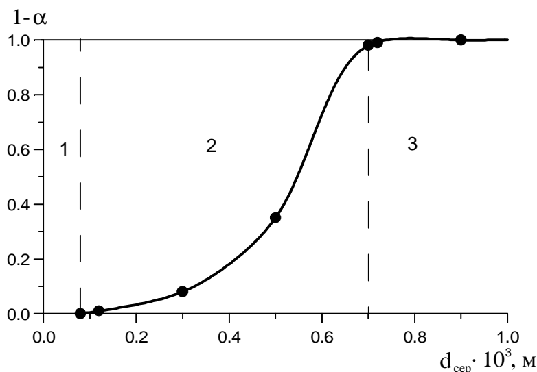
Рис. 2. Вплив розміру подрібнення вихідної сировини на ступінь вилучення олії у вигляді залежності 1 - a = f(d_{\text{cep}})
