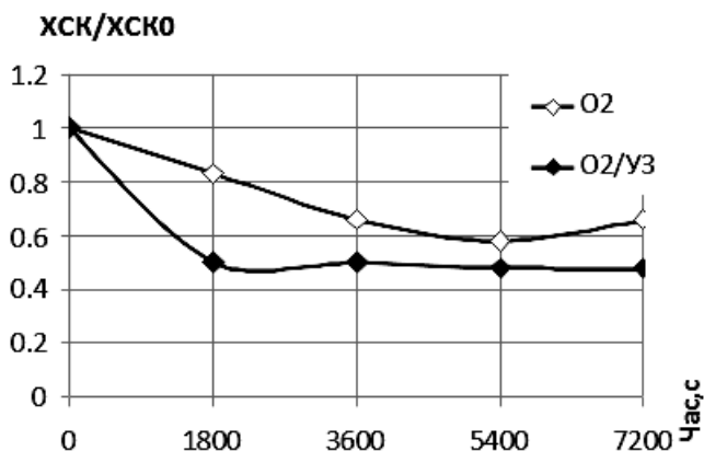
Рис. 2. Залежність відношення X_{СК}/X_{СК0} від часу оброблення стічних вод жиркомбінату в атмосфері кисню за різних умов експерименту
