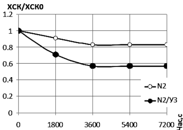
Рис. 1. Залежність відношення X_{СК}/X_{СК0} від часу оброблення стічних вод жиркомбінату в атмосфері азоту за різних умов експерименту
