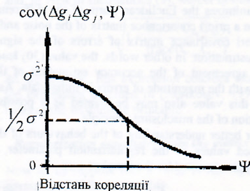
Рис. 1. До визначення коваріаційної функції.
