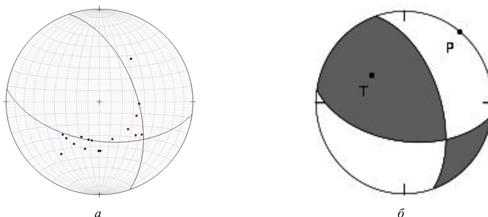
Рис. 1. a – визначення нодальних площин для землетрусу 29.09.2017 за знаками вступів Р-хвиль на 17 станціях; б – відповідний фокальний механізм з квадрантами стиску (темний) і розтягу (світлий) та осями стиску Р і розтягу Т. Параметри механізму наведено в табл. 3 і табл. 4
