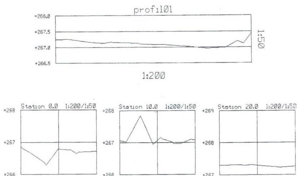
Ryc. 6. Profil podłużny i przekroje poprzeczne („DRAW PROFILE”, „DRAW ALIGNMENT SECTIONS”)
