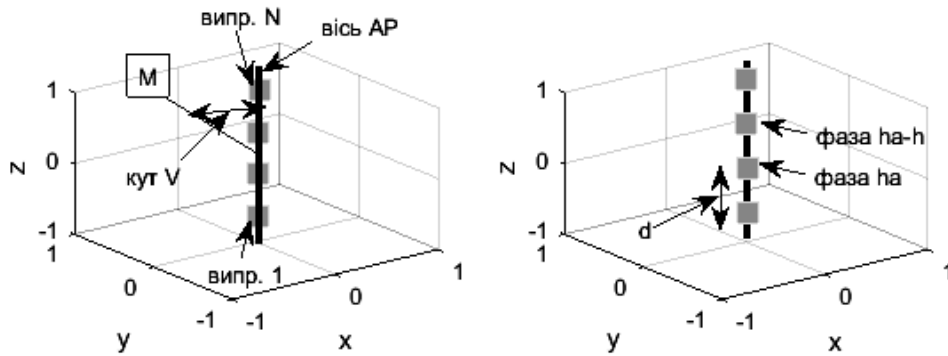
Рис. 1. Будова прямолінійної АР, що містить N випромінювачів
