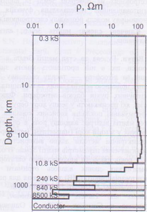
Рис. 2. Одновимірні моделі глибинного геоелектричного розрізу в районі розташування Болгарської геомагнітної обсерваторії Панагюрище (ПАГ).
