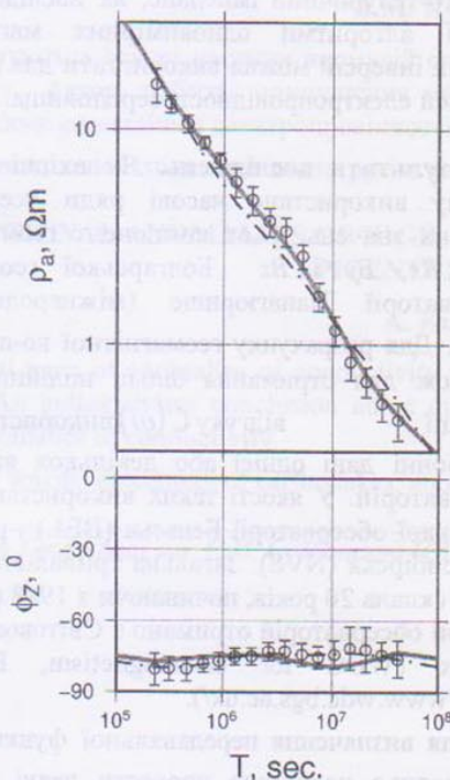
Рис. 1. Глибинні магнітоваріаційні криві позірнього опору та фази імпедансу для обсерваторії ПАГ.
