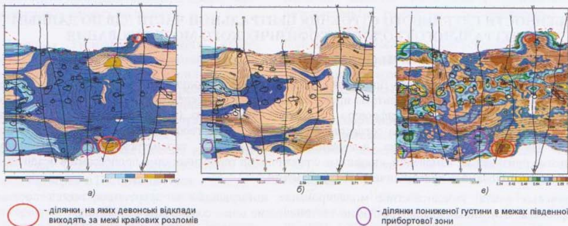
Рис. 2. Перерізи просторової інтегральної моделі у межах верхньодевонських відкладів: а) середньофранський ярус, семилуцький горизонт D_3f_1sm , б) нижньофаменський ярус, задоно-єслєцький горизонт D_3fm_1zd-el , в) верхньофаменський ярус, озерсько-хованський під'ярус D_3fm_3oz-ch
