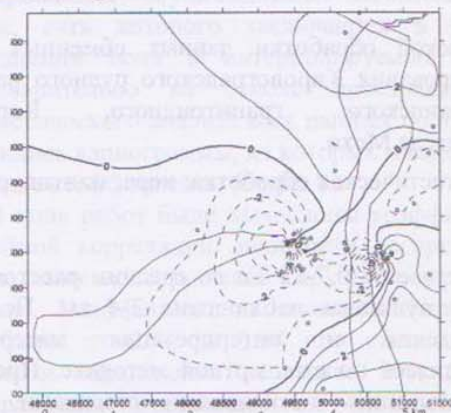
Рис. 5. Карта скоростей относительных вертикальных движений территории ЗАГАЭС-1 за период 2000-2011 гг. по данным ГНСС измерений. Изолинии проведены через 1 мм/год (штрихпунктирные линии отражают опускание, сплошные — подъем)
