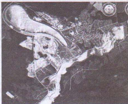
Рис. 2. Космический снимок 2009 г. территории объекта исследований [Image © 2011 GeoEye]
