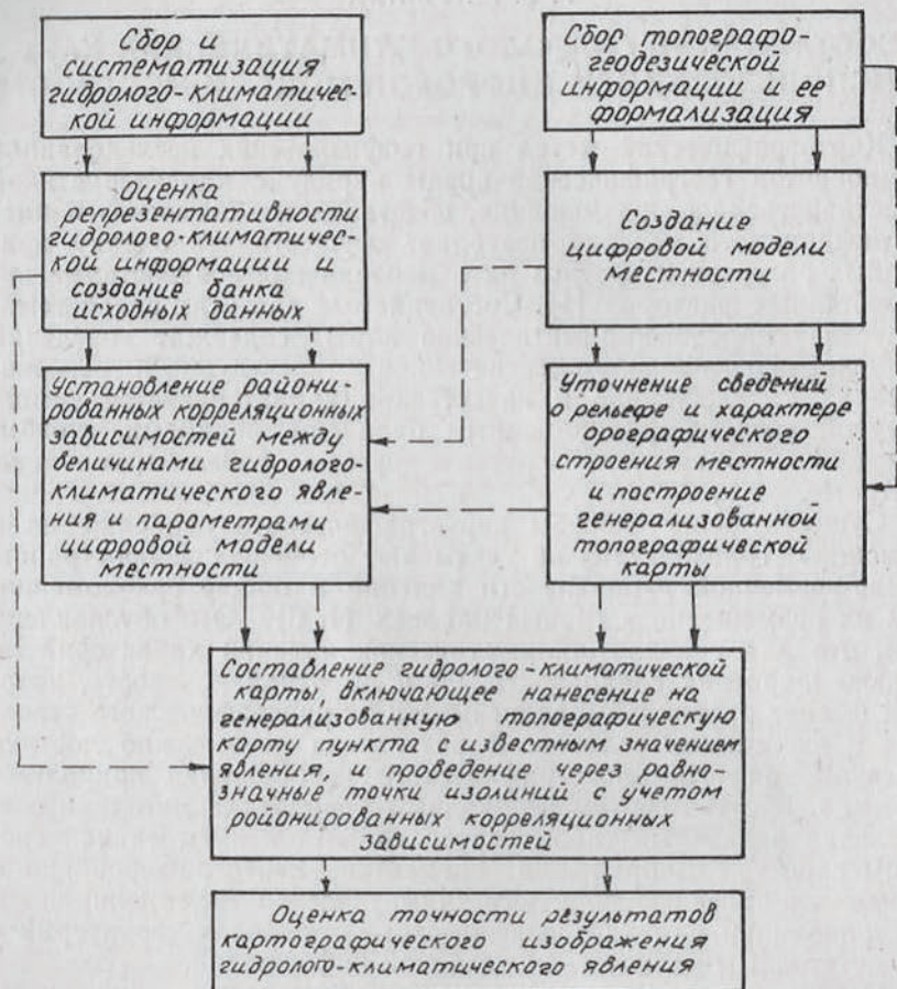
Рис. 1. Блок-схема технологического процесса составления гидролого-климатической карты:
