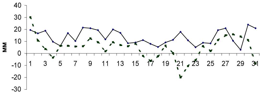
Різниці \Delta d_w за моделлю Saastamoinen
