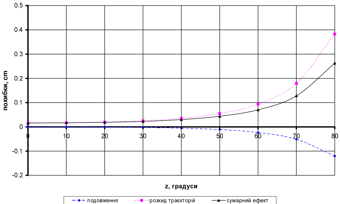
Рис. 2. Рефракційні похибки двочастотного методу для Nm=10^6 \text{ см}^{-3} , f1=1227,46 \text{ МГц} , f2=1575,60 \text{ МГц}
