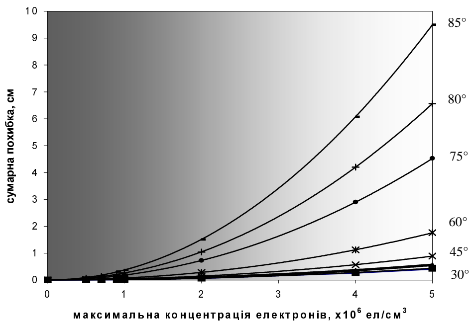
Рис. 3. Залежність сумарної похибки від концентрації електронів на різних зенітних кутах
