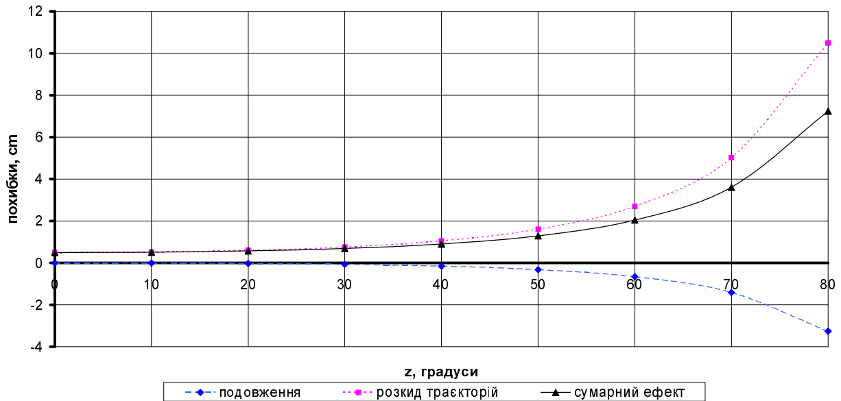
Рис. 1. Рефракційні похибки двочастотного методу для Nm=5 \cdot 10^6 \text{ см}^{-3} , f1=1227,46 \text{ MHz} , f2=1575,60 \text{ MHz}
