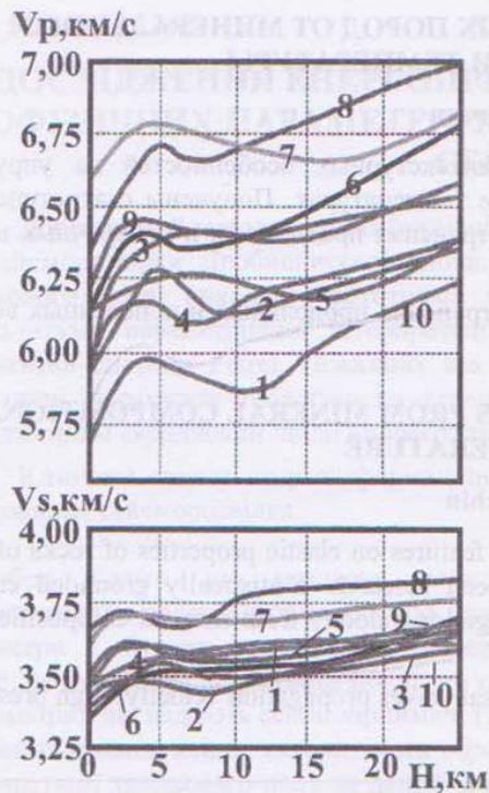
Рис. 1. Зміна з глибиною середніх значень швидкостей V_P і V_S ( V_{P,S}=f(PT)=f(H) ) для різних груп порід УЩ:
