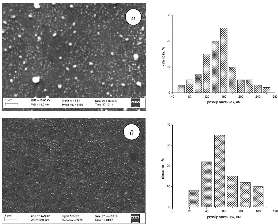
Рис. 2. SEM-зображення поверхні кремнію з осаждением сріблом гальванічним заміщенням у розчинах 0,1\text{M AgNO}_3 (a) та 0,1\text{M} (\text{NH}_4)[\text{Ag}(\text{CN})_2] (b) у DMF і гістограми розподілу частинок осаду за розмірами
