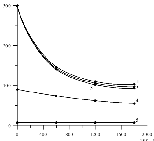
Рис. 2. Вплив природи розчинника та полімеру на ультразвукову деструкцію ( T = 293 К; C_{\text{пол}} = 1 %): I = 5 \cdot 10^4 Вт/м 2 ; розчинник: 1 – ДМСО; 2, 4, 5 – вода; 3 – бутанол; полімер: 1, 2, 3 – ПВП; 4 – ПВС; 5 – ПЕГ
