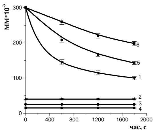
Рис. 1. Зміна молекулярної маси ПВП під дією ультразвуку ( T = 293 К; C_{\text{ПВП}} = 1 %): потужність УЗ, I \cdot 10^4 , Вт/м 2 : 1...4 – 5; 5 – 3; 6 – 1; M_{\text{ПВП}} \cdot 10^{-3} : 1, 5, 6 – 300; 2 – 44; 3 – 28; 4 – 12
