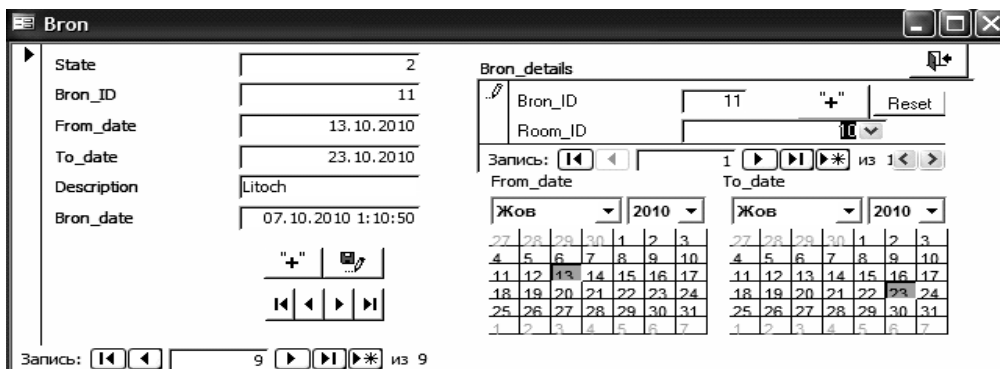
Рис. 6. Форма Bron
