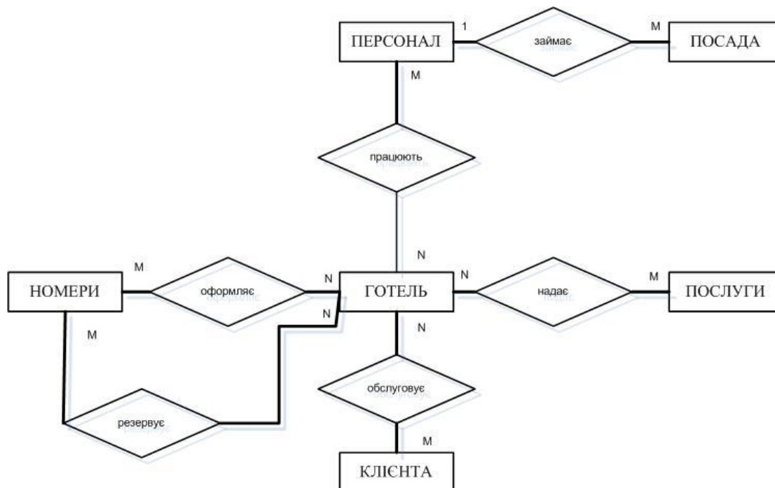
Рис. 3. ER- діаграма предметної області діяльності готелю
