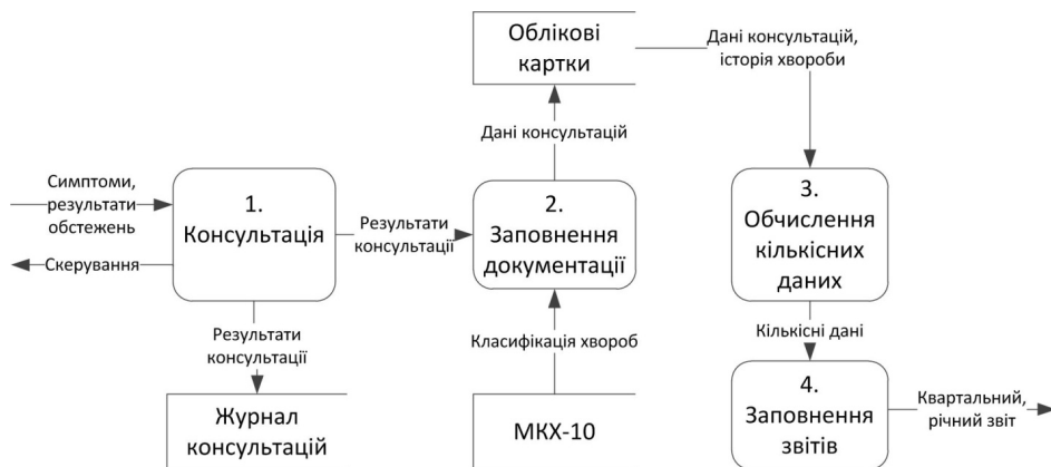
Рис. 4. Діаграма потоків даних предметної області
