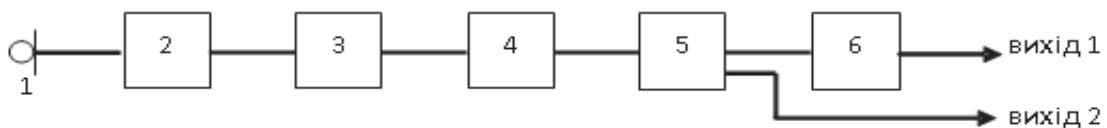
Рис. 5. Структурна схема пристрою для вимірювання параметрів акустичної емісії: 1 – в'єзоперетворювач; 2 – попередній підсилювач; 3 – блок фільтрів; 4 – основний підсилювач; 5 – дискримінатор; 6 – детектор
