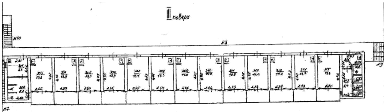
Рис. 3. План третього поверху спального корпусу в "Політехніку-3" в с. Коблево
