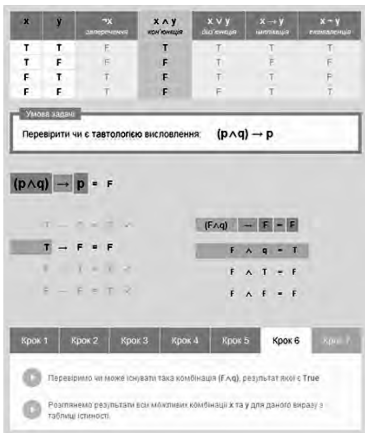
Рис. 7. Інтерфейс веб-аплікації
