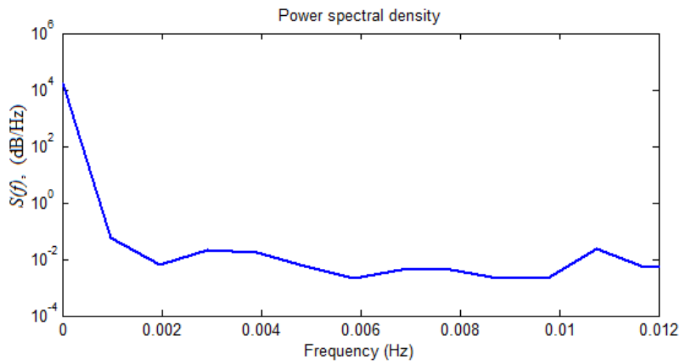
Рис. 3. Енергетичний спектр флуктуацій вимірюваного опору
