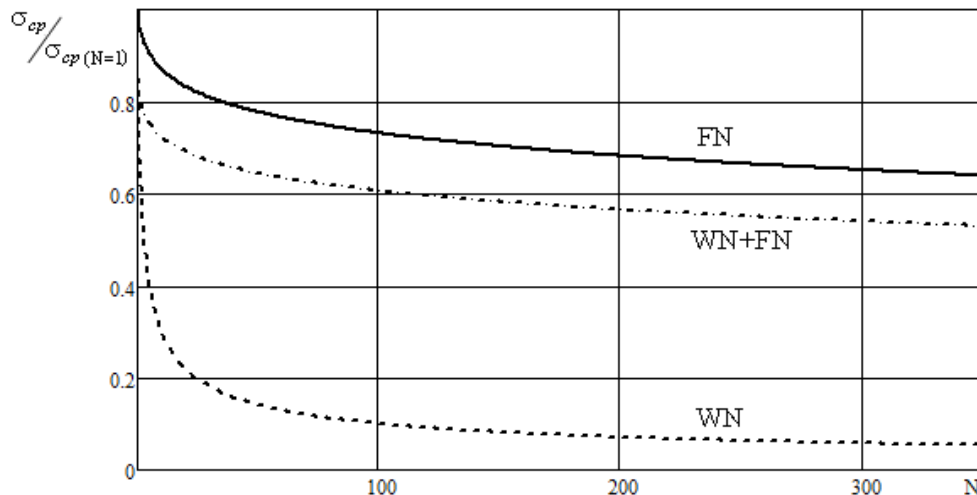
Рис. 4. Залежність нормованого стандартного відхилення результатів вимірювань від кількості вимірювань якщо WN – “білий” шум; FN – фліккер-шум; WN+FN – “білий” шум і фліккер-шум
