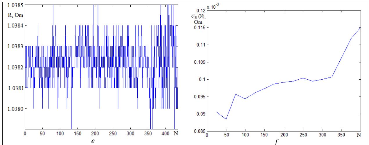
Рис. 1. Результати статистичних вимірювань електричного опору резистора R та залежності стандартного відхилення результатів вимірювань від кількості вимірювань \sigma_R(N)
