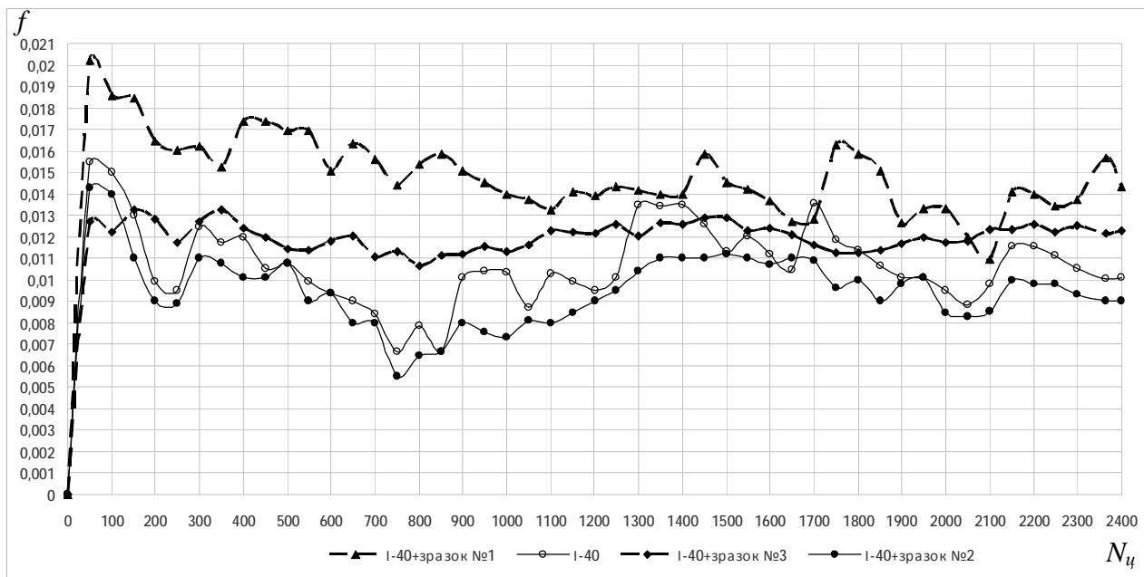
Рис. 2. Коефіцієнт тертя оливи I-40A у композиції з добавками (температура мастильного середовища 90 °C)
