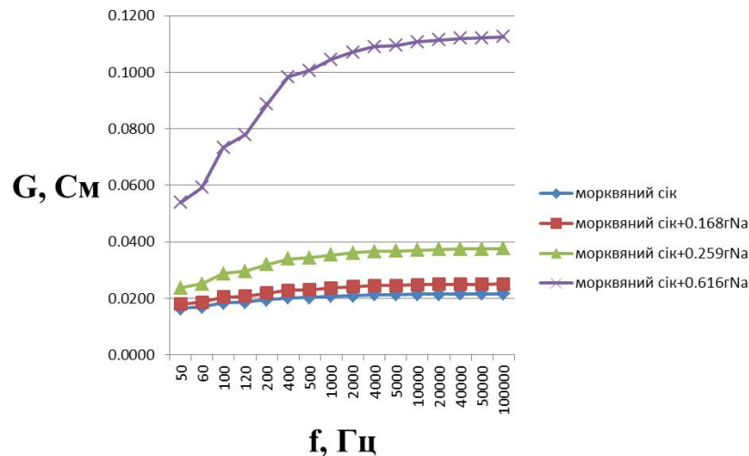
Рис. 3. Залежність активної складової G провідності від концентрації Na_2SO_4 у модельній рідині
