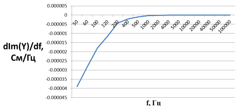
Рис. 6. Графік залежності швидкості зміни реактивної складової B провідності від частоти
