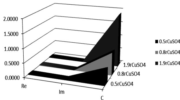
Рис. 11. Залежність складових електропровідності модельної рідини на частоті 1000 Гц від вмісту домішок Fig. 11. Dependence of components of conductivity of a model liquid at a frequency of 1000 Hz on the content of impurities
