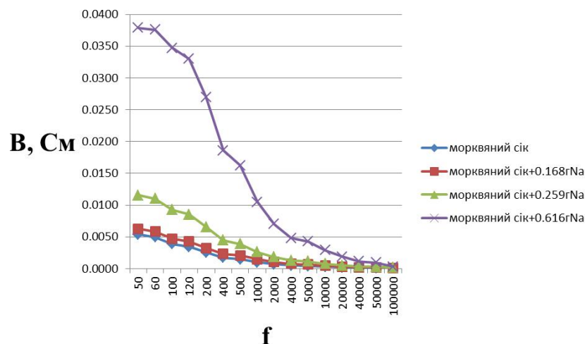
Рис. 4. Залежність реактивної складової B провідності від концентрації Na_2SO_4 у модельній рідині
