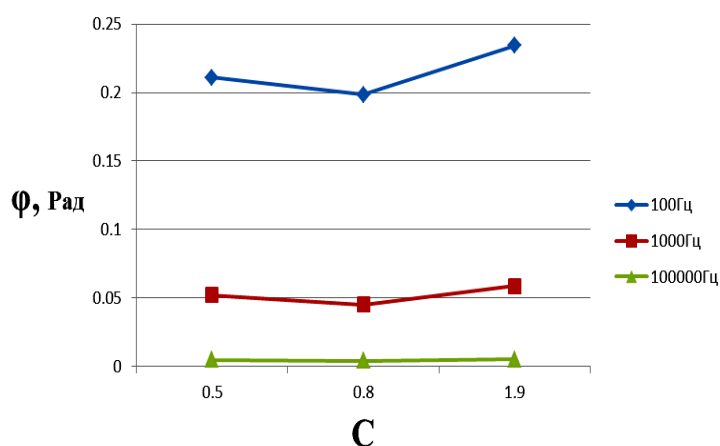
Рис. 9. Залежність фази адмітансу від концентрації Cu
