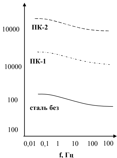
Рис. 4. Імпедансна залежність для сталевих зразків з полікарбоксилатними покриттями після 7 діб витримки у вологій камері за 40°С
