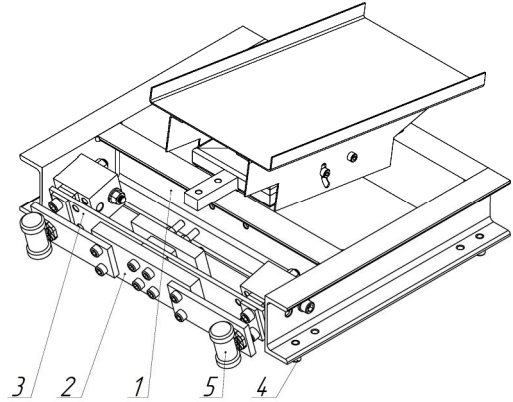
Рис. 4. Двомасова вібраційна машина Fig. 4. The two-mass vibration machine
