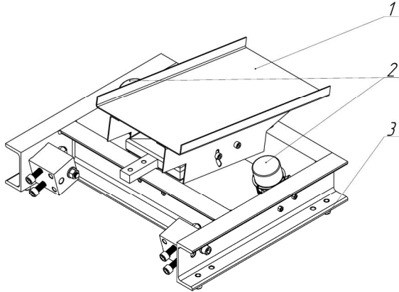
Рис. 3. Одномасова вібраційна машина Fig. 3. The single-mass vibration machine
