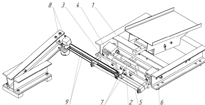
Рис. 5. Тримасова вібраційна машина
