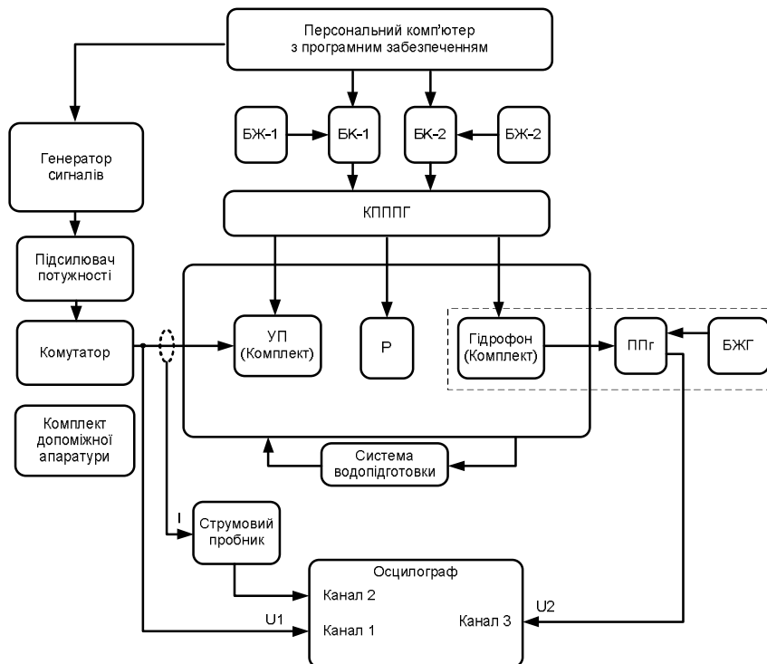
Рис. 2. Функціональна схема еталона: КПППГ – координатно-поворотний пристрій позиціонування гідрофонів; БЖ-1, БЖ-2 – блоки живлення; БК-1 та БК-2 – блоки керування; БЖГ – блок живлення гідрофона; ППГ – попередній підсилювач гідрофона; УП – ультразвуковий перетворювач; Р – рефлектор
