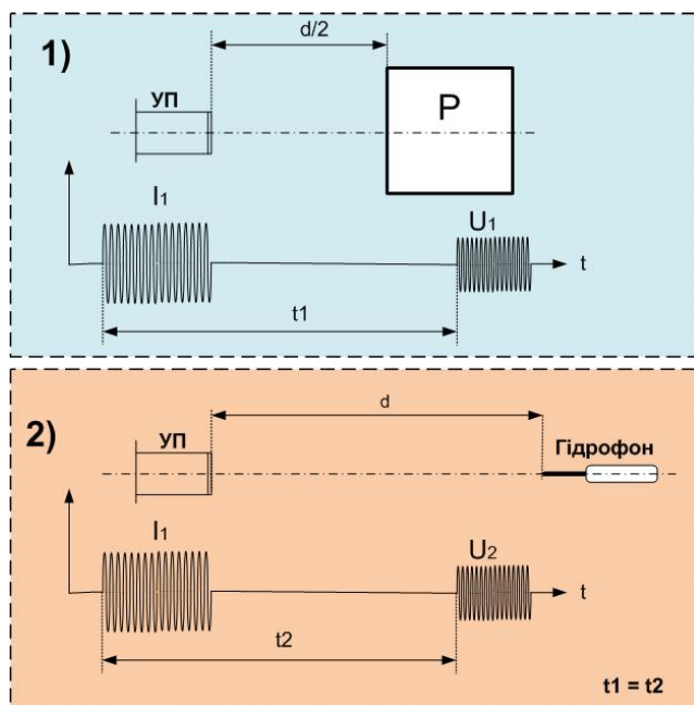
Рис. 1. Визначення чутливості гідрофона методом взаємності із двома перетворювачами: Р – рефлектор, УП – допоміжний перетворювач, t_1 , t_2 – час між випромінюванням і прийнятим сигналом на першому і другому етапі вимірювання, який пропорційний до вимірювальної відстані d
