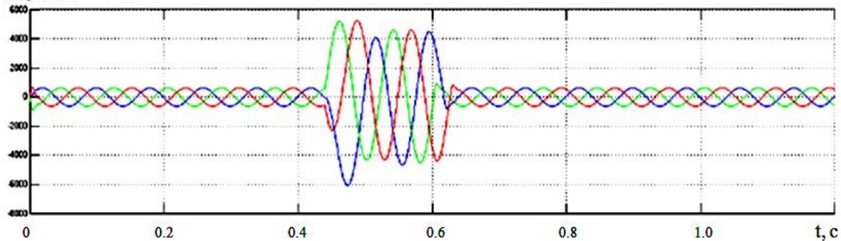
Рис.8. Комп'ютерні осцилограми напруги та струму в режимі трифазного короткого замикання
