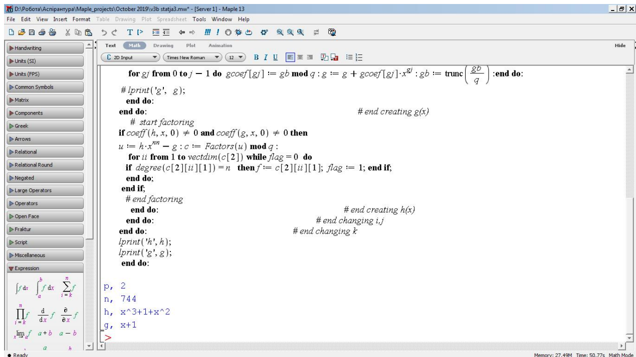
Рис. 3. Вікно середовища Maple з обчисленими поліномами g(x) та h(x)
