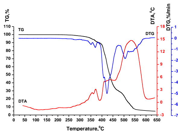
Рис. 4. Термограма зразка 3 (зістарений бітум 10 год)
