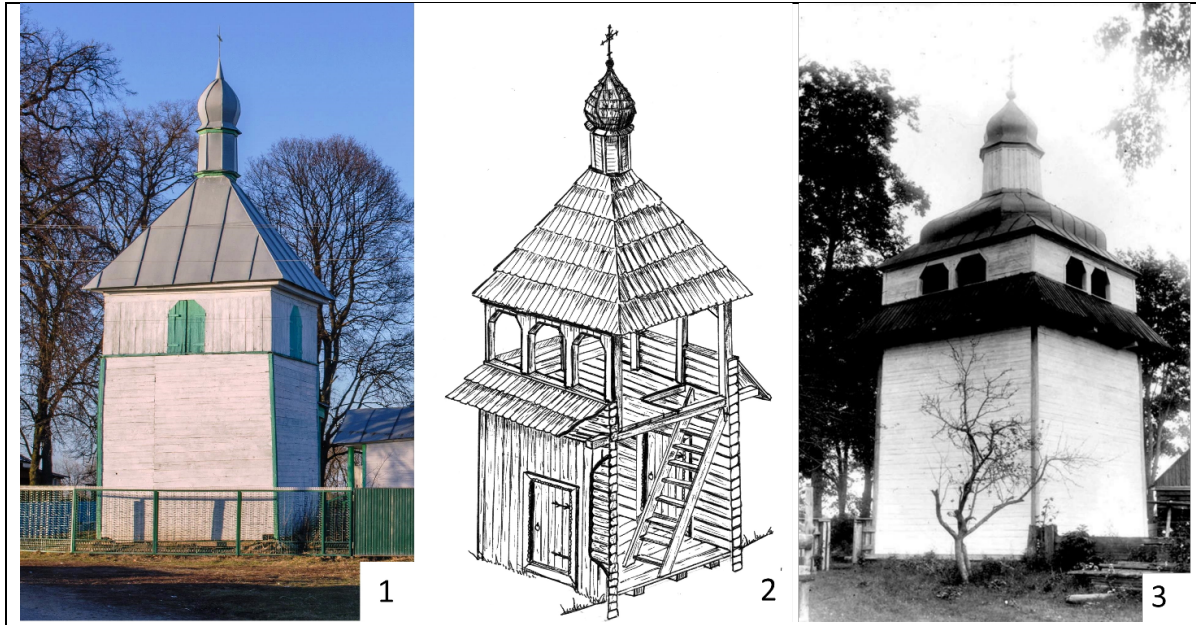
Рис. 4. Дзвіниці кінця XVII–XVIII ст.: Новий Білоус, сучасний вигляд (світлина 2016 р.); 2. Варіант реконструкції дзвіниці в Новому Білоусу станом на XVIII ст. (малюнок автора); 3. Пакуль, світлина 1908 р.
