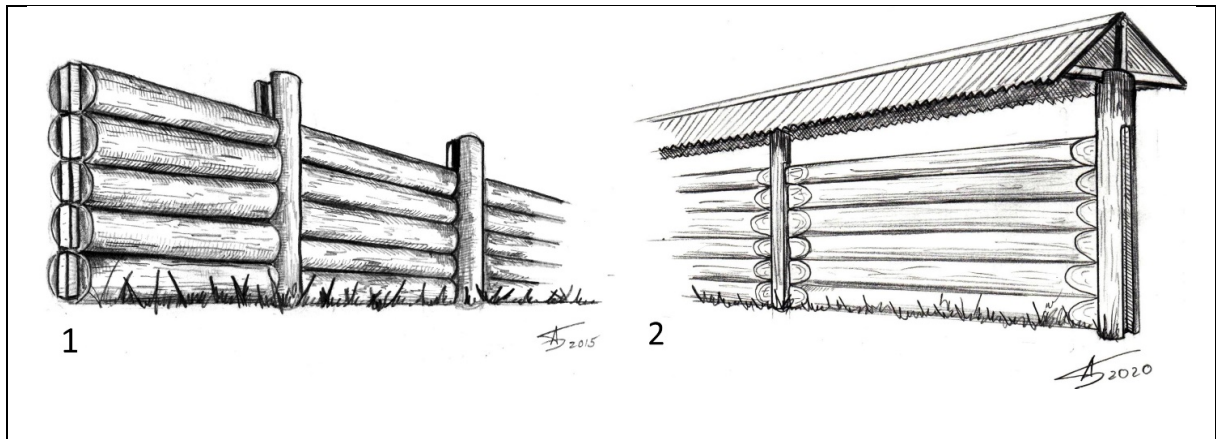
Рис. 1. Паркан «в забор» за етнографічними даними Чернігівщини: 1. простий тип «забору»; 2. «забор» з дашком (малюнки автора)
