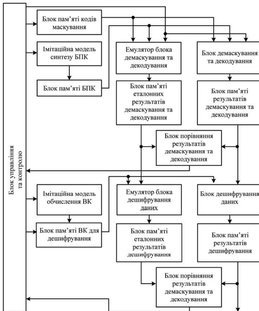
Рис. 3. Інформаційна модель відлагодження й тестування блоків декодування, демаскування та дешифрування даних / Information model for debugging and testing blocks of decoding, unmasking and decryption of data
