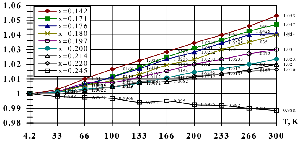
R(T)/R(4.2K)
