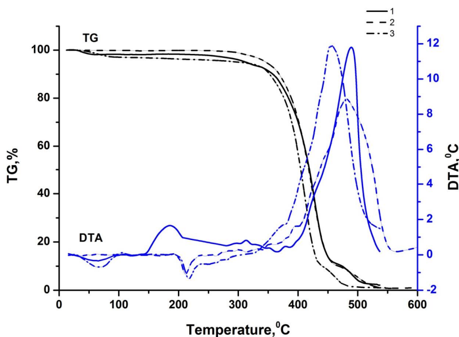
Рис. 1. Зведені криві ТГ і ДТА зразків нанокompозитів ПА6/МПС = 90/10 м. ч., одержаних з форміатного розчину: 1 – нанокompозит ПА6/МПС; 2 – нанокompозит, термооброблений за 250 °С; 3 – нанокompозит, оброблений на капілярному пластометрі за температури 230 °С
