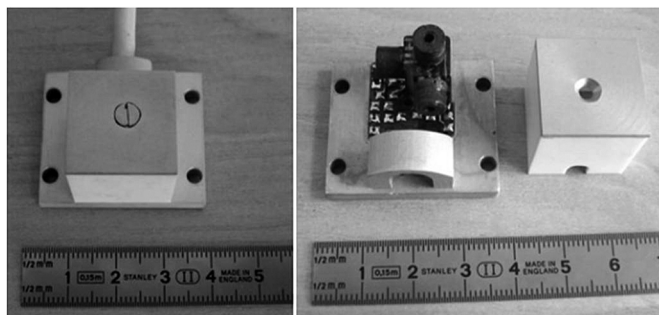
Рис. 5. Конструкція 3D-зонда
