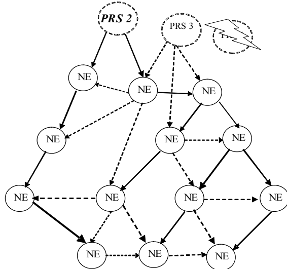
Рис. 2. Традиційний спосіб резервування у разі аварії PRS 1
