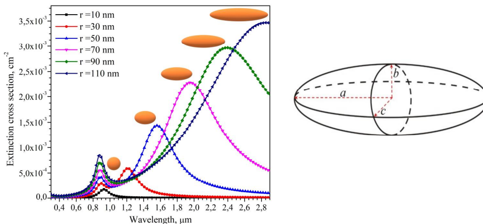
Рис. 2. Спектри екстинкції еліпсоїдних наночастинок CuS, які поміщені в середовище з показником заломлення 1,0003, зі сталим розміром півосей b = c = 10 нм та змінною довжиною півосі a
