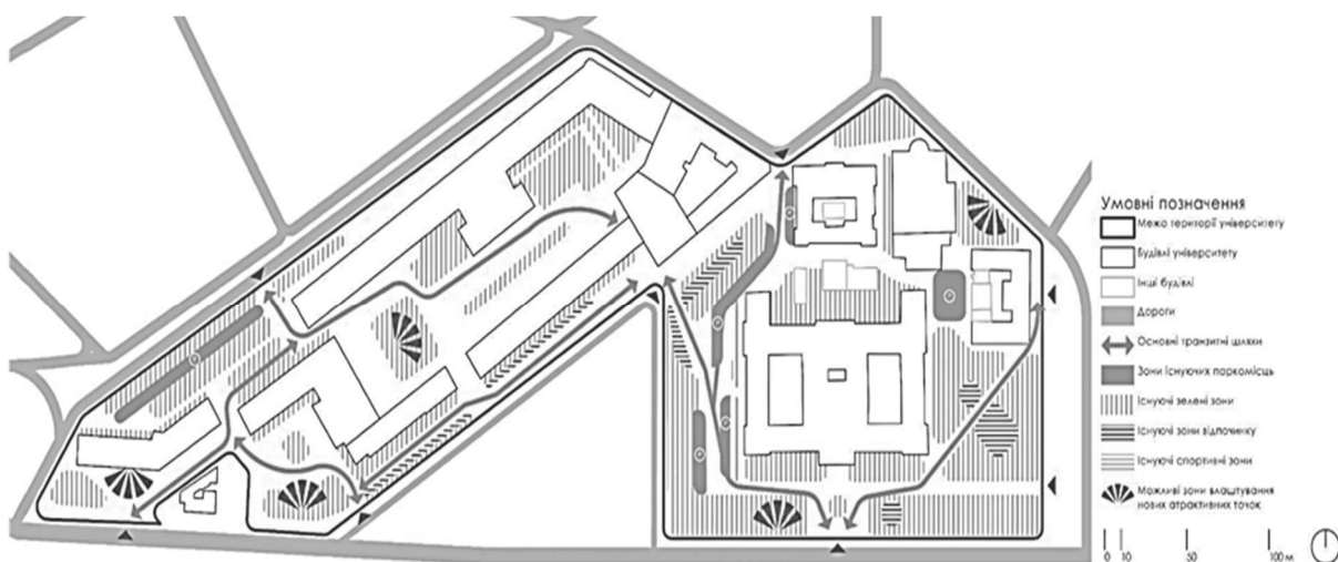
Рис. 1. Схема наявного стану території Національного університету "Львівська політехніка" (схему розробила А. Нікуліна)
