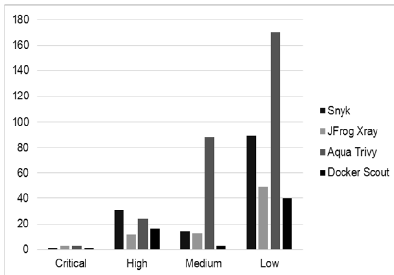
Рис. 3. Середні значення кількості знайдених вразливостей кожного типу
