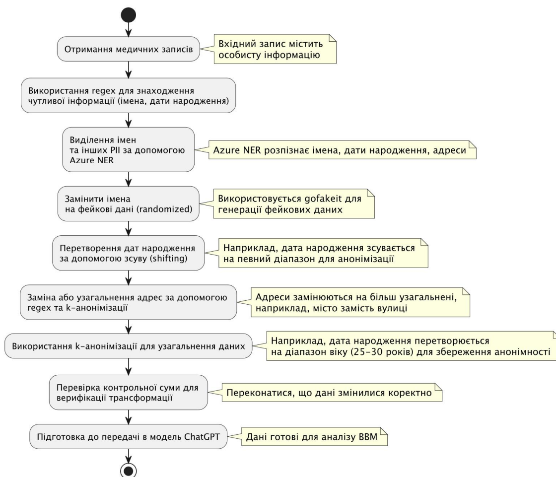
Рис. 2. Схема роботи процесу анонімізації
