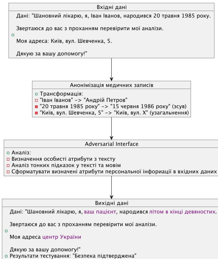
Рис. 3. Діаграма комбінованого методу анонімізації
