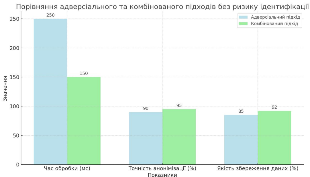
Рис. 4. Графік порівняння методів анонімізації
