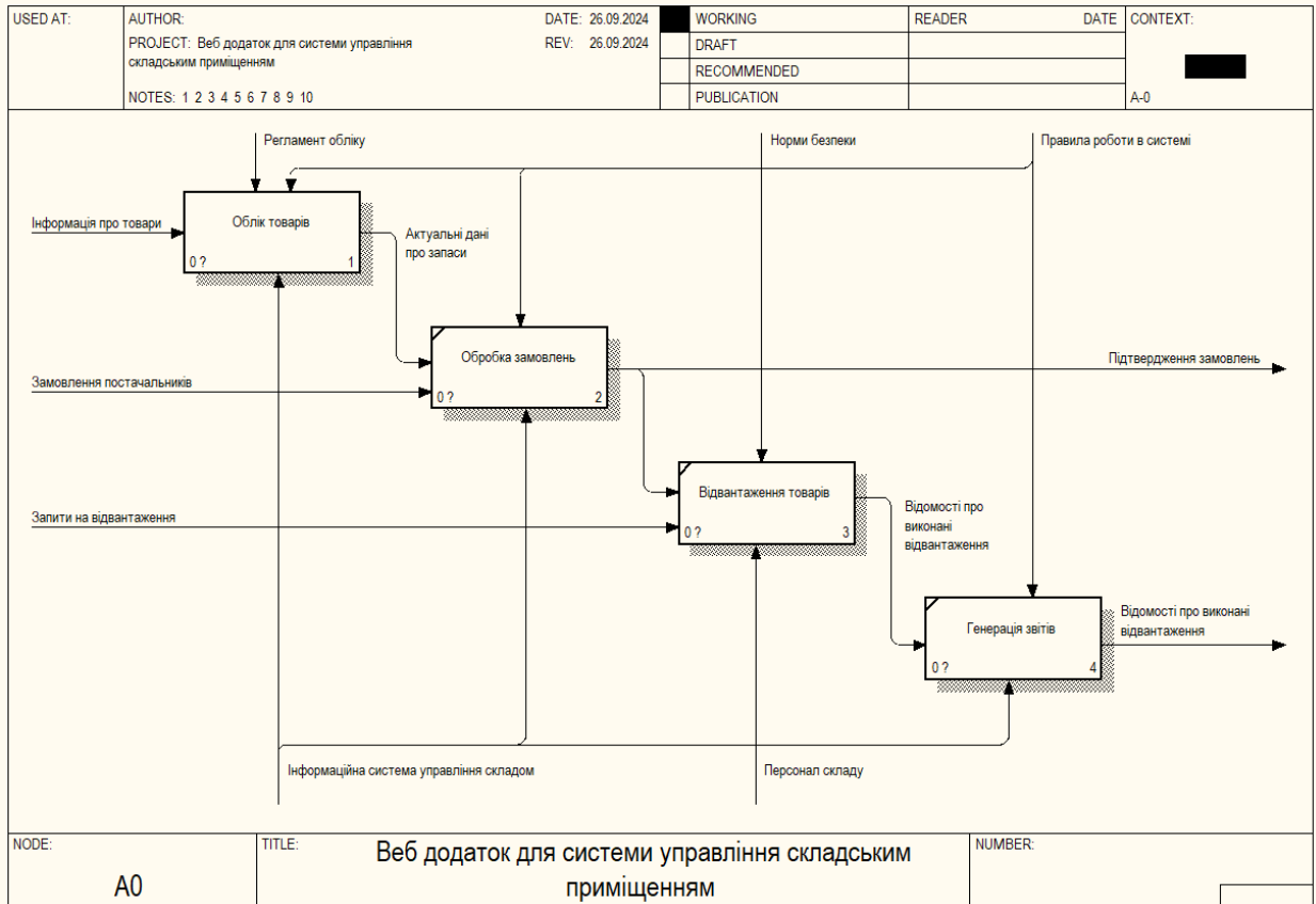
Рис. 2. Діаграма першого рівня декомпозиції системи управління складським приміщенням.
