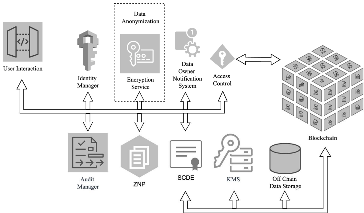
Рис. 1. Модель анонімізації даних
