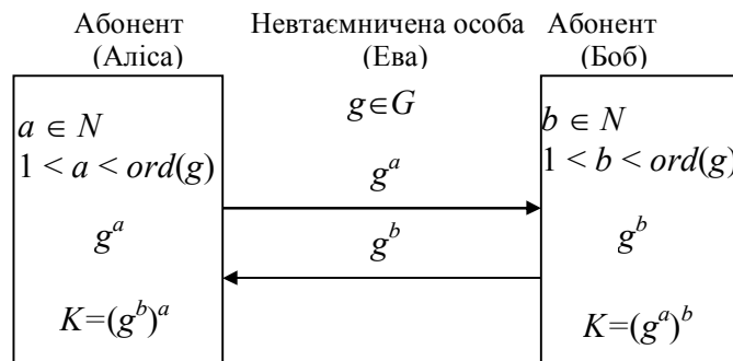
Рис. 2. Протокол Діфі-Хелмана
