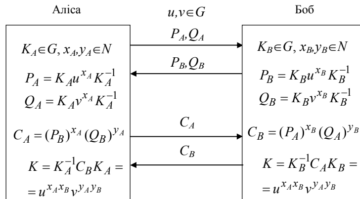
Рис. 4. Протокол Лізами-Ромеро
