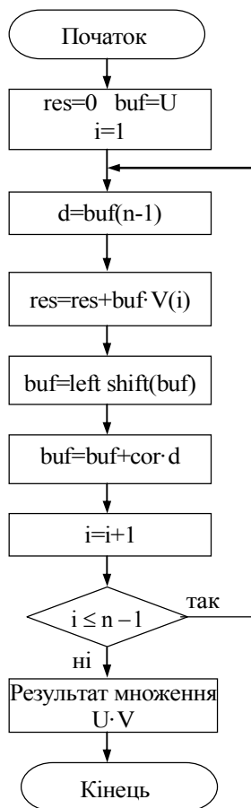
Рис. 1. Блок-схема множення елементів скінченного поля
