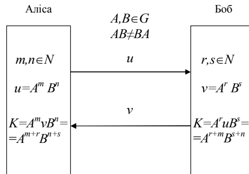
Рис. 3. Протокол Стікеля
