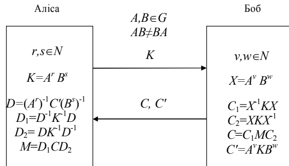
Рис. 5. Криптосистема Канвал-Алі
