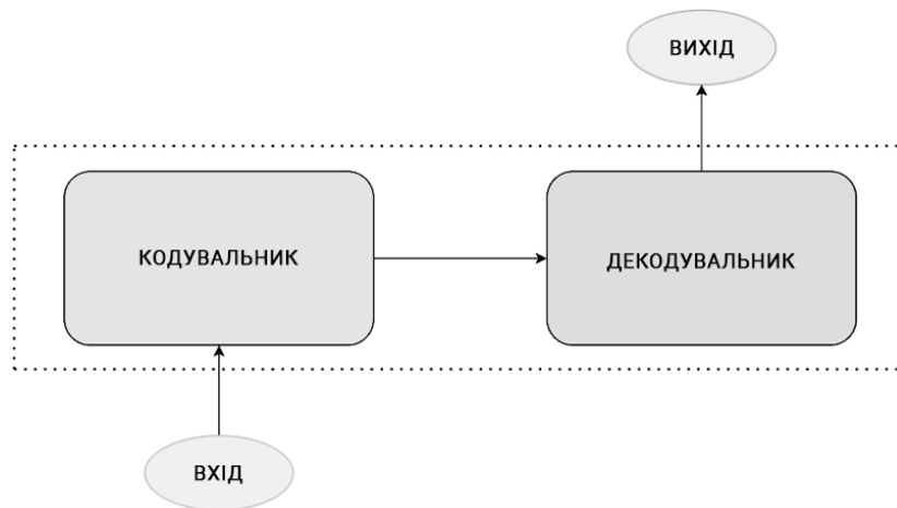
Рис. 1. Архітектура трансформера
