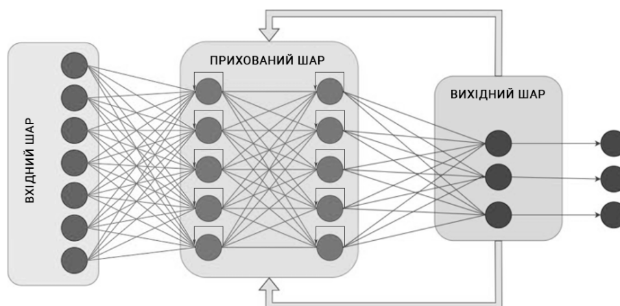
Рис. 2. Архітектура рекурентної нейронної мережі
