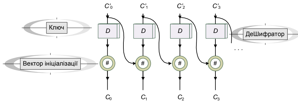
Рис.4. Схема дешифрування
