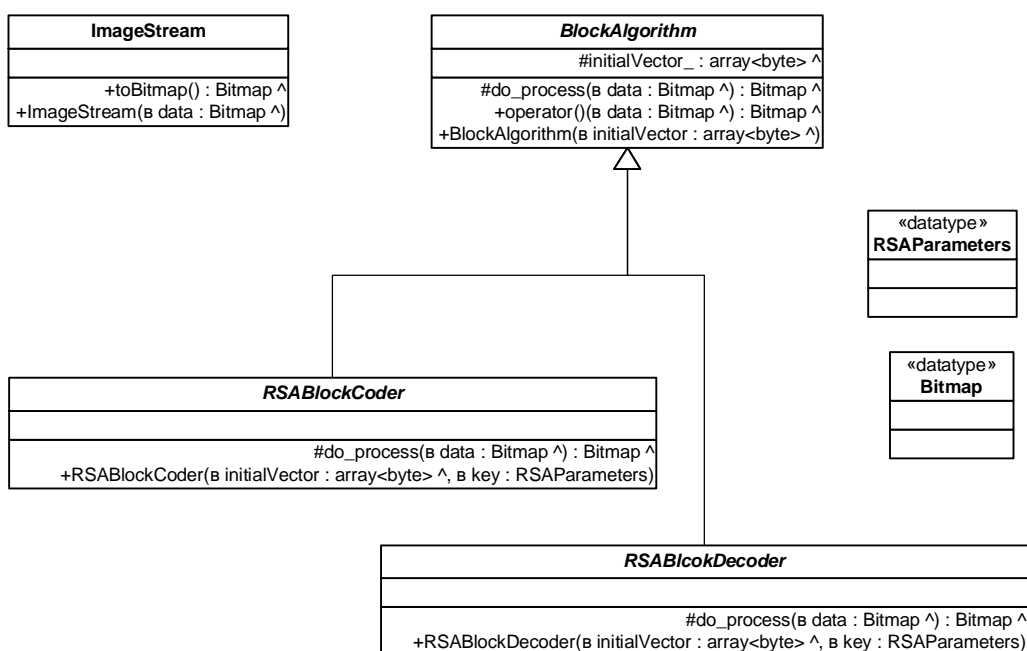
Рис. 7. Діаграма класів
