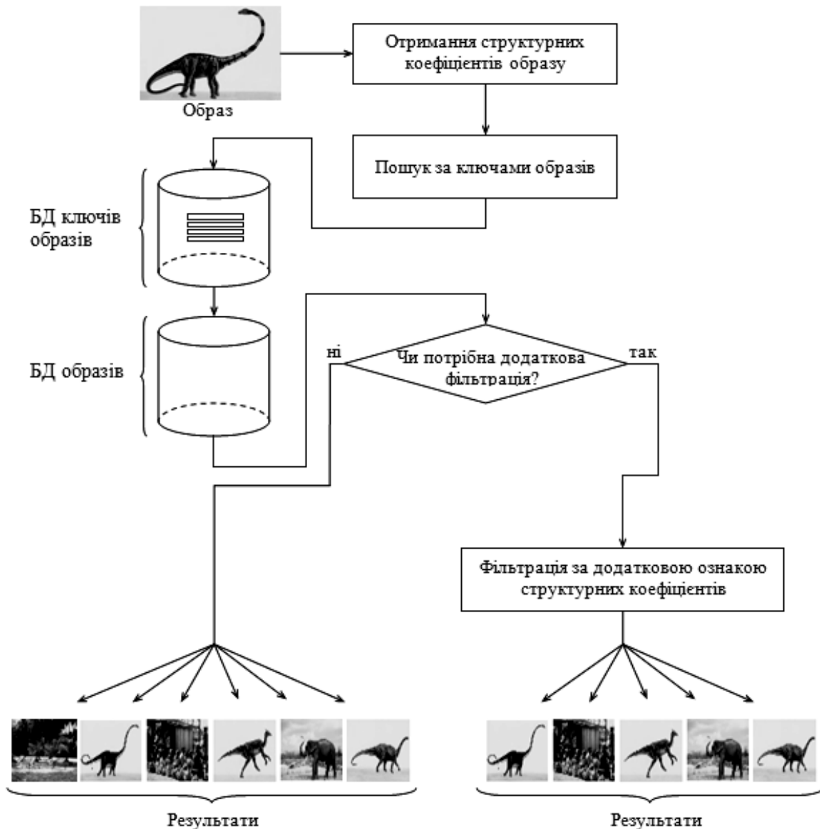
Рис. 4. Схема процесу пошуку образів
