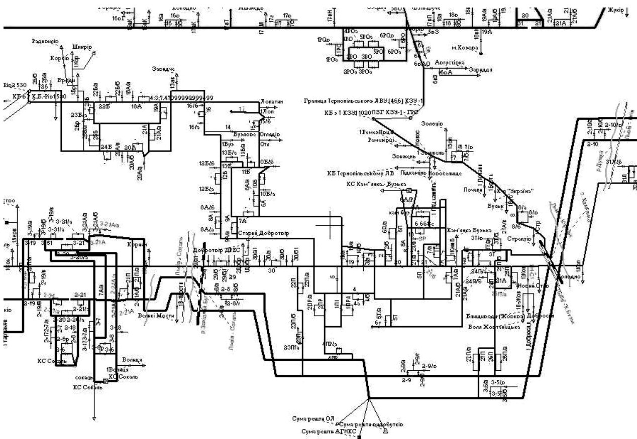
Рис. 4. Технологічна схема
