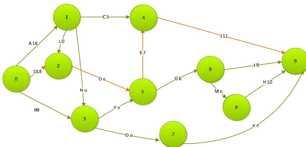
Рис. 5. Представлення проєкту у вигляді мережі типу “робота–дуга”
