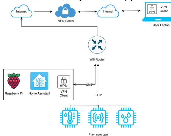
Рис. 7. Схема підключення до кіберфізичної системи через VPN
